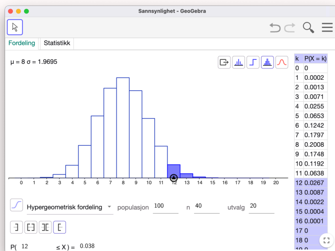
Figur 3: Hypergeometrisk hypotesetest i GeoGebra til oppgave 2-2
