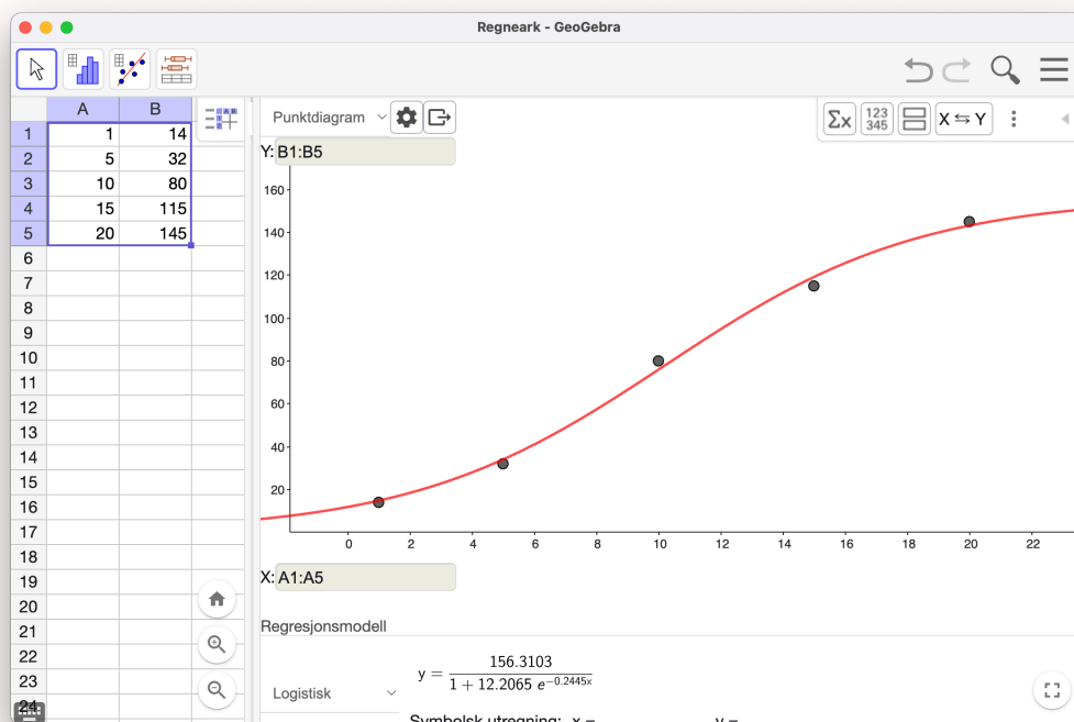
Figur 1: Regresjon av logistisk funksjon i GeoGebra
